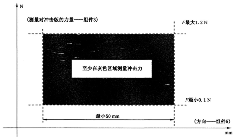
图 11 冲击力分布
